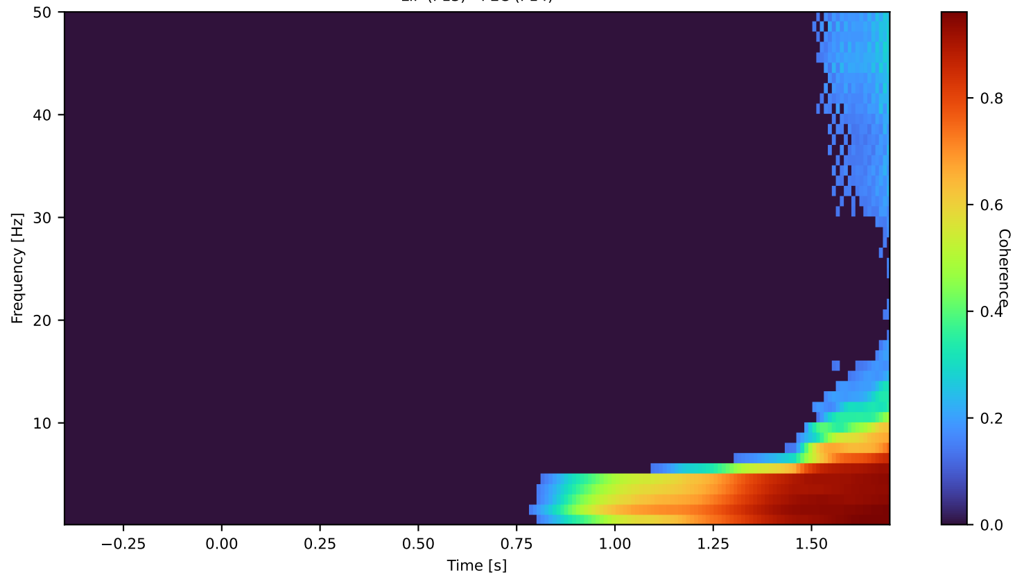
LIP (P13) - PEC (P14)
